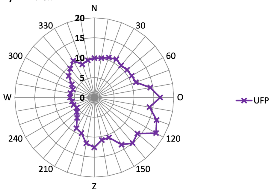
Figuur 3. Pollutieroos van UFP (paarse lijn met kruizen) voor meetstation Sluiskil, eerste half jaar 2024. De as in de grafiek geeft de gemiddelde concentratie per windrichting van 10° weer in duizend deeltjes/cm 3 .
