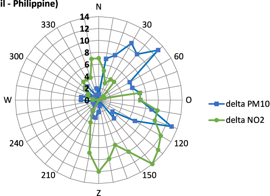
Figuur 4. Pollutierozen van de verschilconcentraties voor \text{PM}_{10} (blauwe lijn met vierkanten) en \text{NO}_2 (groene lijn met cirkels), eerste half jaar 2024. De verschilconcentraties zijn berekend door de concentraties op station Philippine van station Sluiskil af te trekken. De as in de grafiek geeft de gemiddelde concentratie per windrichting van 10^\circ weer in \mu\text{g}/\text{m}^3 .
