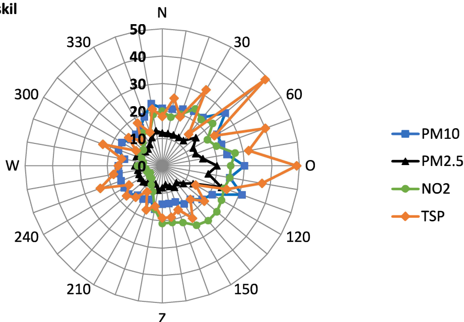
Figuur 2. Pollutierozen van TSP (oranje lijn met ruiten), PM 10 (blauwe lijn met vierkanten), PM 2.5 (zwarte lijn met driehoeken) en NO 2 (groene lijn met cirkels) voor meetstation Sluiskil, voor het eerste half jaar 2024. De as in de grafiek geeft de gemiddelde concentratie in \mu\text{g}/\text{m}^3 per windrichting van 10° weer.
