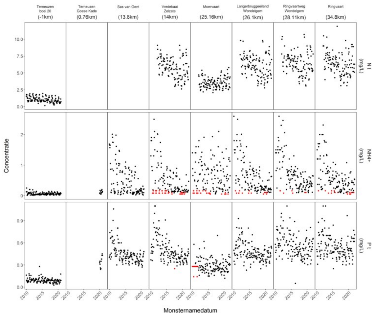
Figuur 9: Verloop van de nutriënten doorheen het studiegebied en aangrenzende waterlichamen met aanduiding van de metingen waarbij de concentratie niet bepaald kon worden door de detectielimiet (ROOD)
