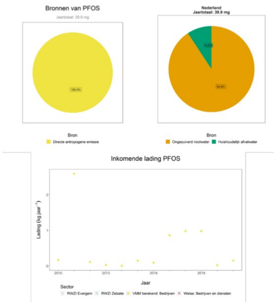
Figuur 75: PFOS – emissie naar KGT: de gemiddelde jaarlijkse lading naar het volledige kanaal (LINKSBOVEN), detail van de Directe antropogene emissie voor Nederland (RECHTSBOVEN) en de door de VMM berekende vrachten voor de bedrijven (ONDER).
