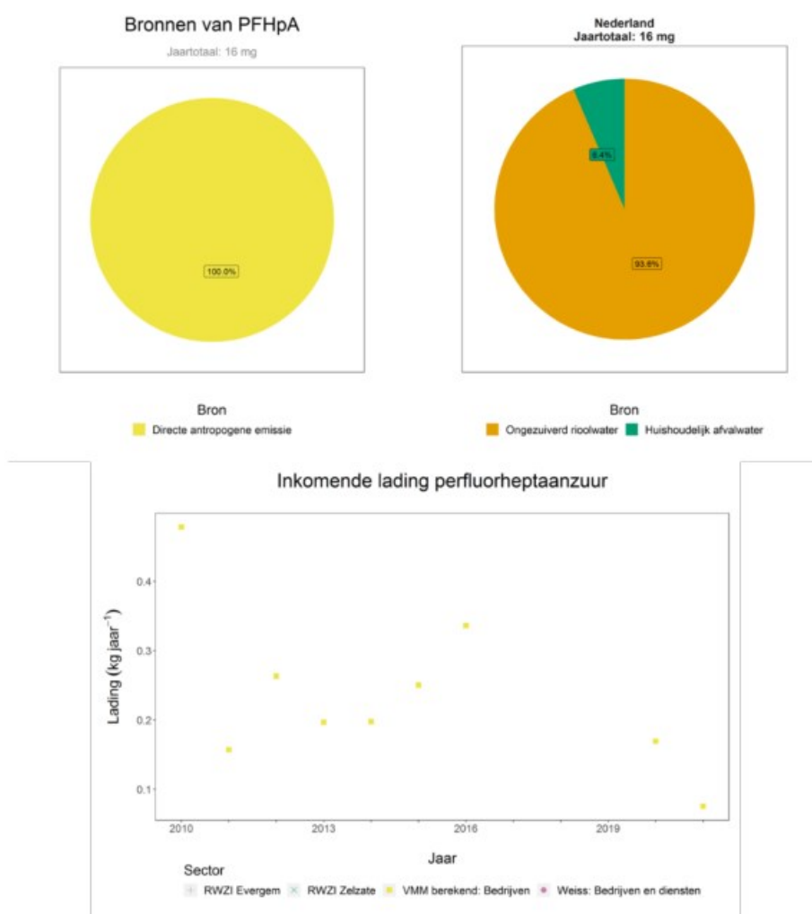
Figuur 64: PFHpA – emissie naar KGT: de gemiddelde jaarlijkse lading naar het volledige kanaal (LINKSBOVEN), detail van de Directe antropogene emissie voor Nederland (RECHTSBOVEN) en de door de VMM berekende vrachten voor de bedrijven (ONDER).
