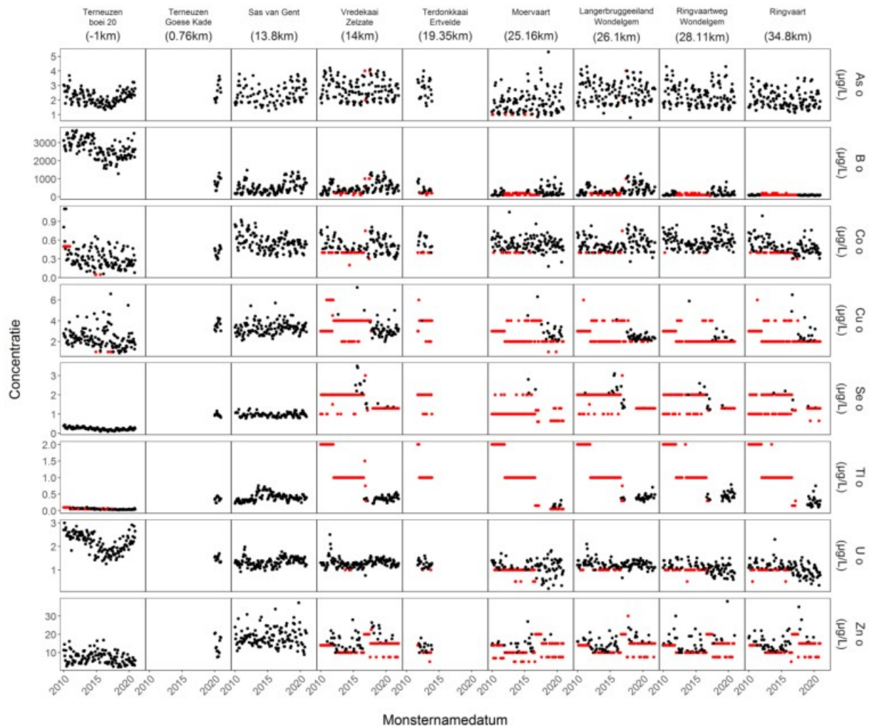
Figuur 19: Verloop van metalen (opgeloste concentratie) doorheen het studiegebied en aangrenzende waterlichamen met aanduiding van de metingen waarbij de concentratie niet bepaald kon worden door de detectielimiet (ROOD)
