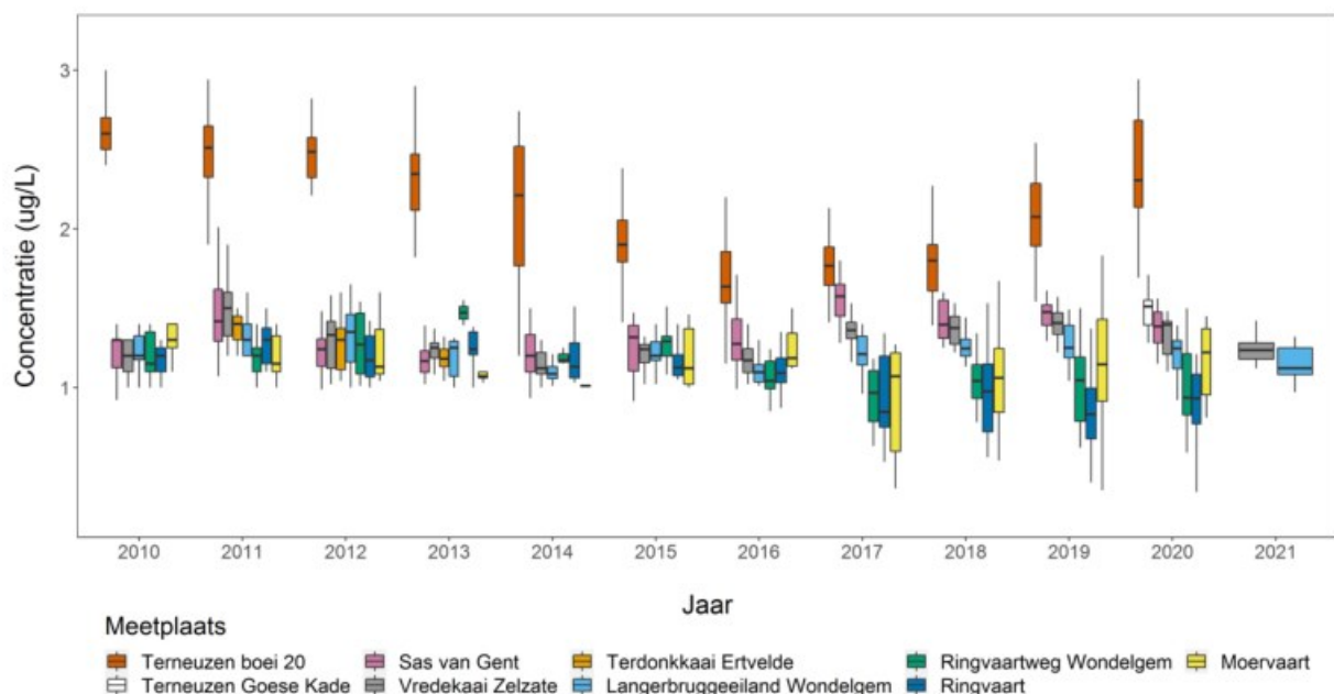
Concentratie U o langs meetpunten
