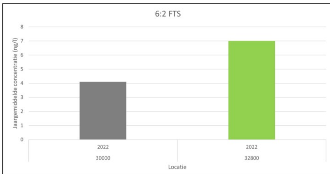
Figuur 77: Jaargemiddelde concentratie (2022) van 6:2 FTS voor de meetlocaties Vredekaai Zelzate (30000) en Rodenhuizeakaai Desteldonk (32800) o.b.v. DOV databank.
