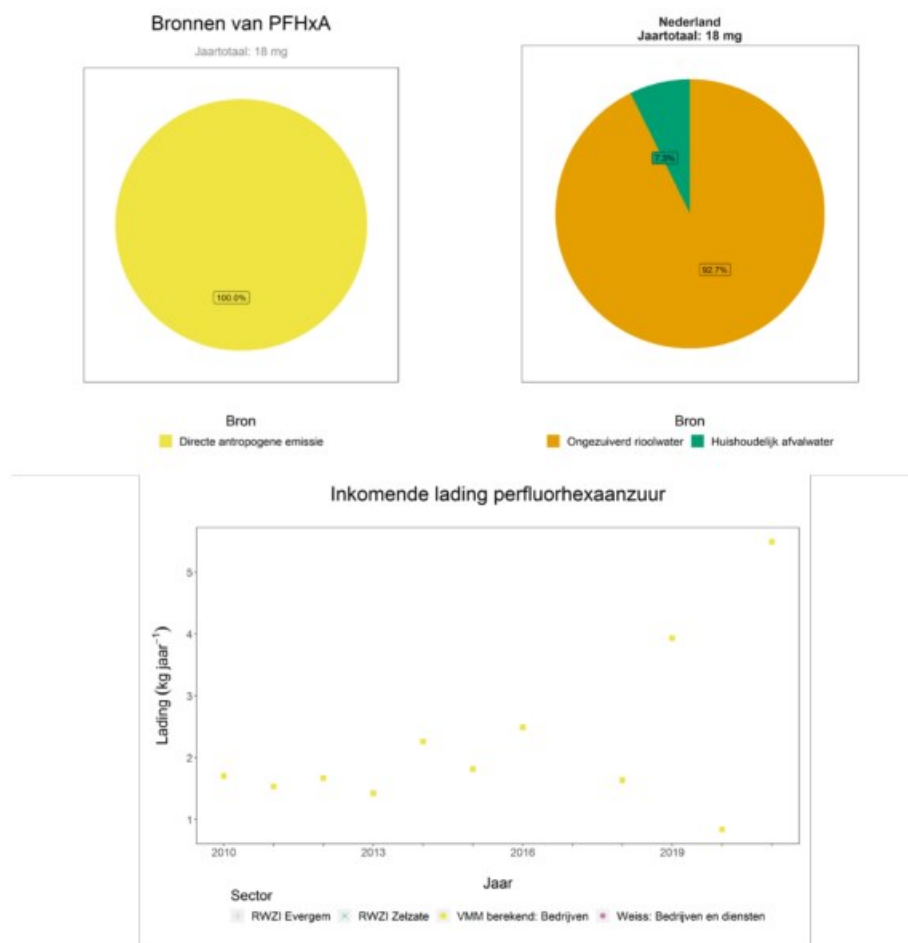
Figuur 62: PFHxA – emissie naar KGT: de gemiddelde jaarlijkse lading naar het volledige kanaal (LINKSBOVEN), detail van de Directe antropogene emissie voor Nederland (RECHTSBOVEN) en de door de VMM berekende vrachten voor de bedrijven (ONDER).
