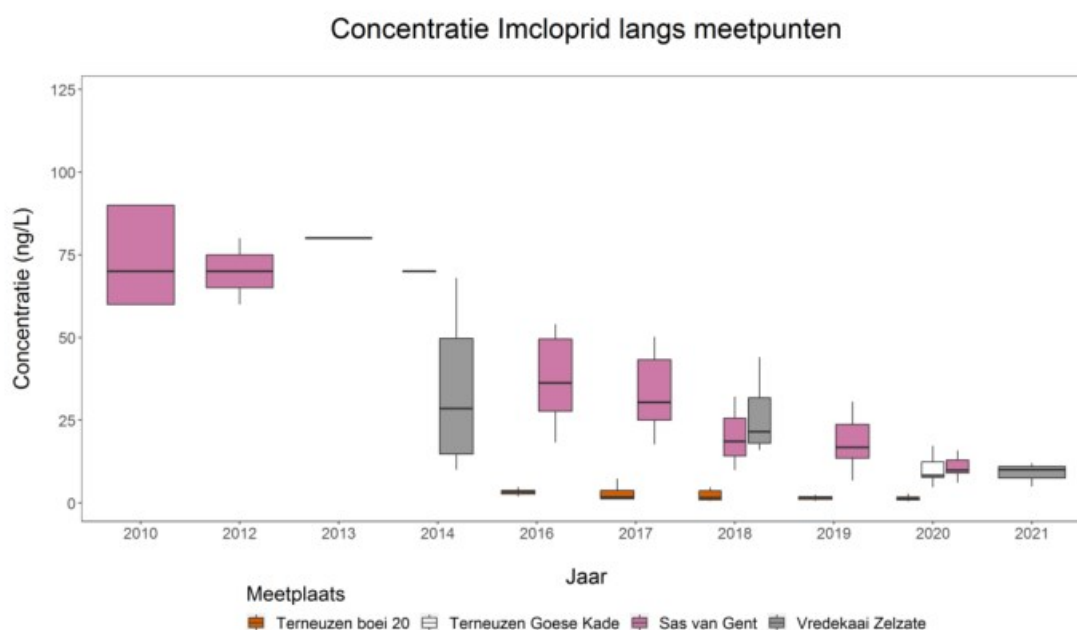
Figuur 80: Imidacloprid – Verloop gemeten concentratie doorheen studiegebied.
