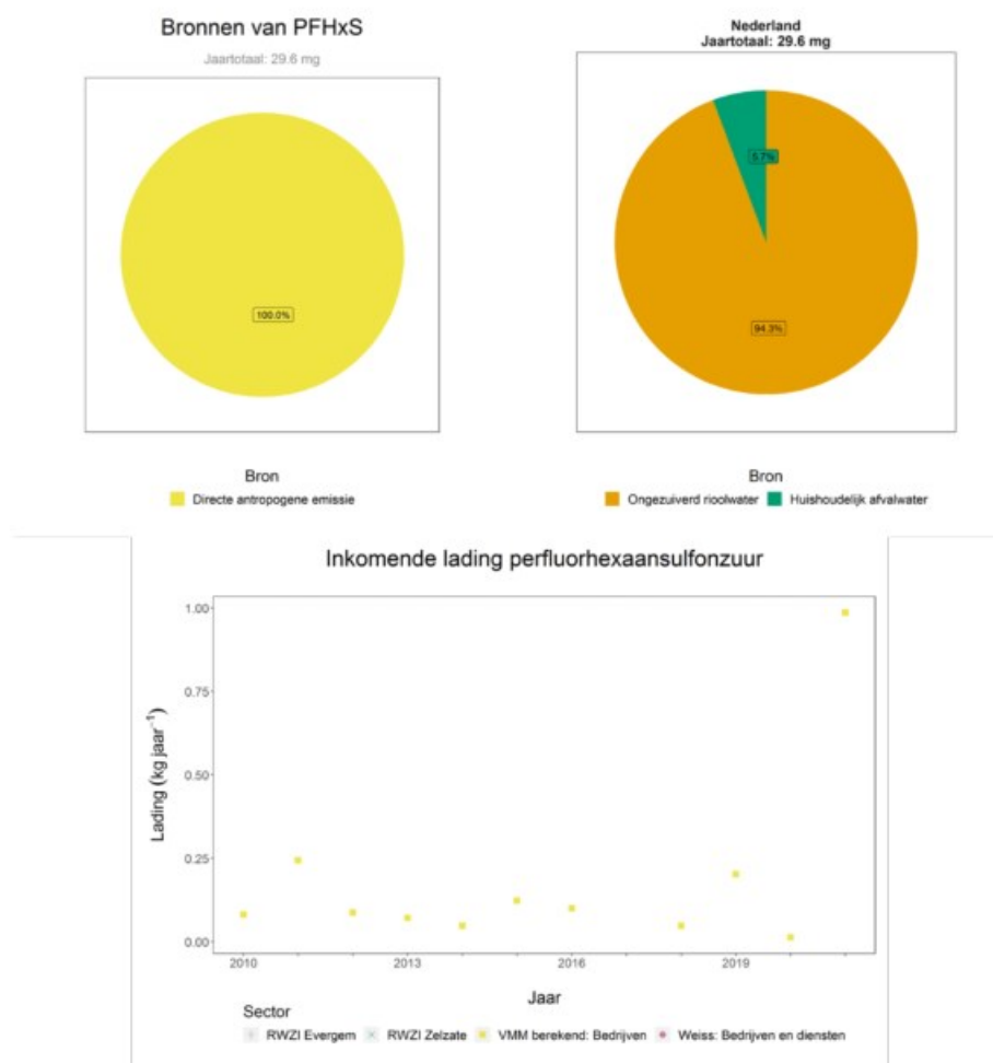
Figuur 72: PFHxS – emissie naar KGT: de gemiddelde jaarlijkse lading naar het volledige kanaal (LINKSBOVEN), detail van de Directe antropogene emissie voor Nederland (RECHTSBOVEN) en de door de VMM berekende vrachten voor de bedrijven (ONDER).
