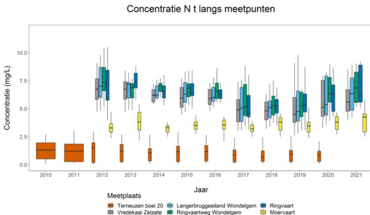
Figuur 10: N tot – Verloop gemeten concentratie doorheen studiegebied.
