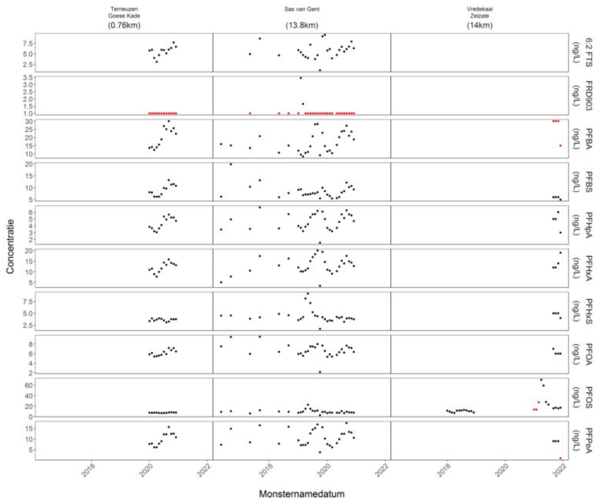
Figuur 54: Verloop van PFAS doorheen het studiegebied en aangrenzende waterlichamen met aanduiding van de metingen waarbij de concentratie niet bepaald kon worden door de detectielimiet (ROOD)
