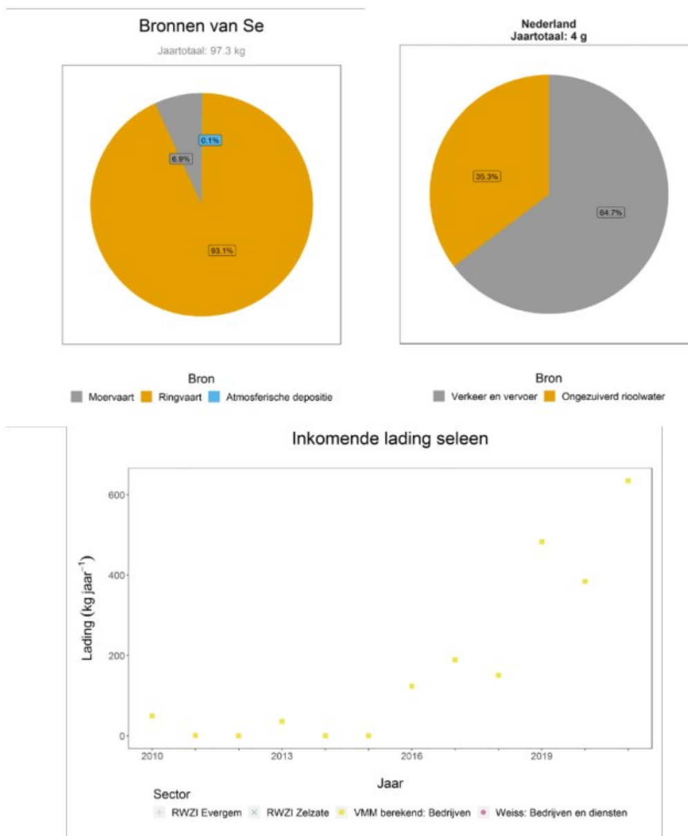
Figuur 33: Seleen Totaal – emissie naar KGT: de gemiddelde jaarlijkse lading naar het volledige kanaal – Merk op: de influx via bovenafvoer is een overschatting t.g.v. de detectielimiet in België (LINKSBOVEN), detail van de Directe antropogene emissie voor Nederland (RECHTSBOVEN) en de door de VMM berekende vrachten voor de bedrijven (ONDER).
