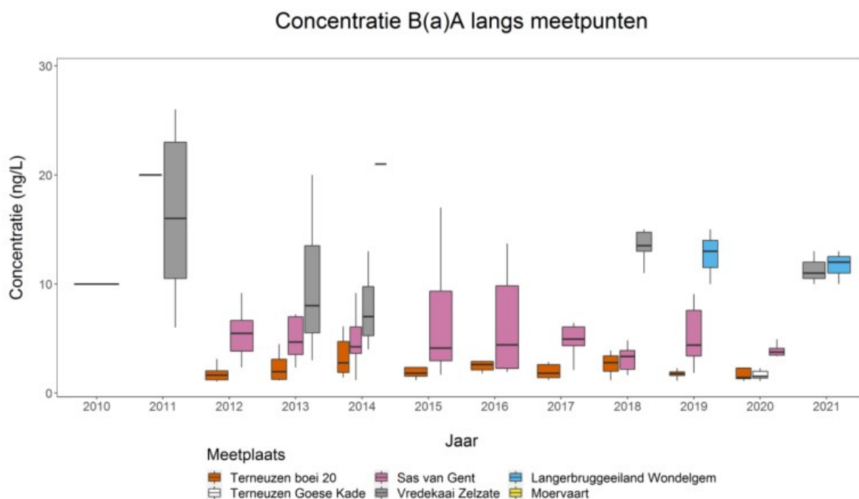
Figuur 45: B(a)A – Verloop gemeten concentratie doorheen studiegebied.
