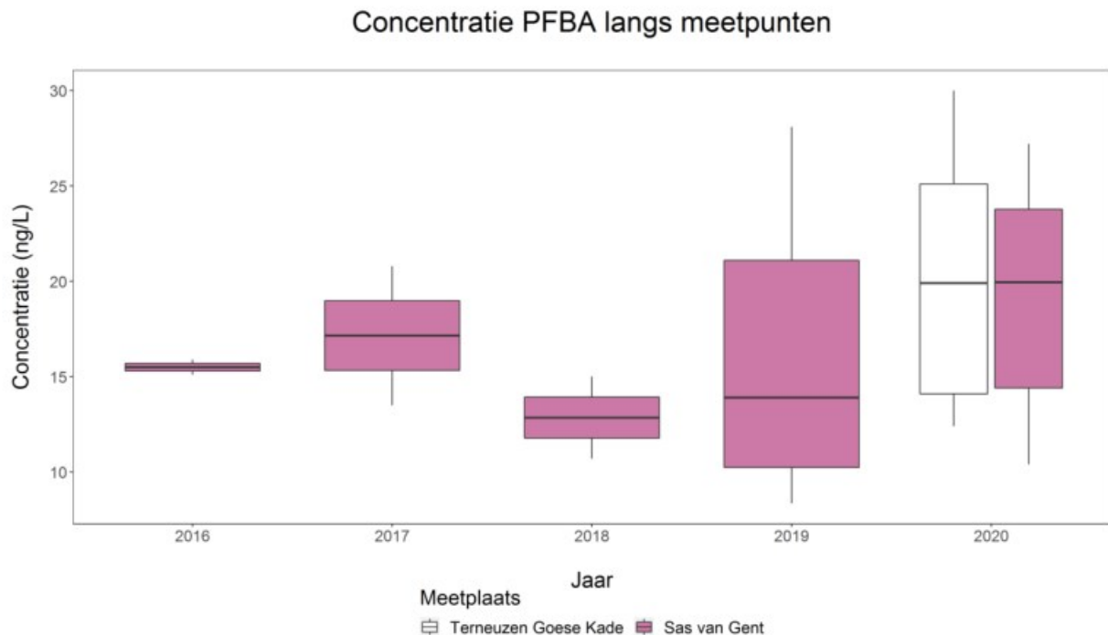
Figuur 55: PFBA – Verloop gemeten concentratie doorheen studiegebied.
