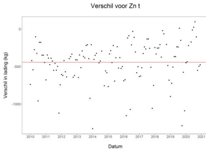
Figuur 43: Zink Totaal – Verschil tussen de berekende maandelijkse emissie naar het KGT en het uit de gemeten concentratie geschatte totaalgewicht aanwezig in KGT tijdens dezelfde maand (Zwarte punten). De rode lijn geeft de gemiddelde bias weer over alle punten.
