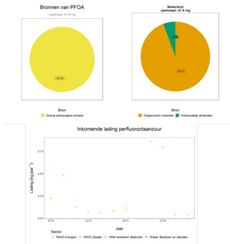
Figuur 66: PFOA – emissie naar KGT: de gemiddelde jaarlijkse lading naar het volledige kanaal (LINKSBOVEN) en de door de VMM berekende vrachten voor de bedrijven (RECHTS).
