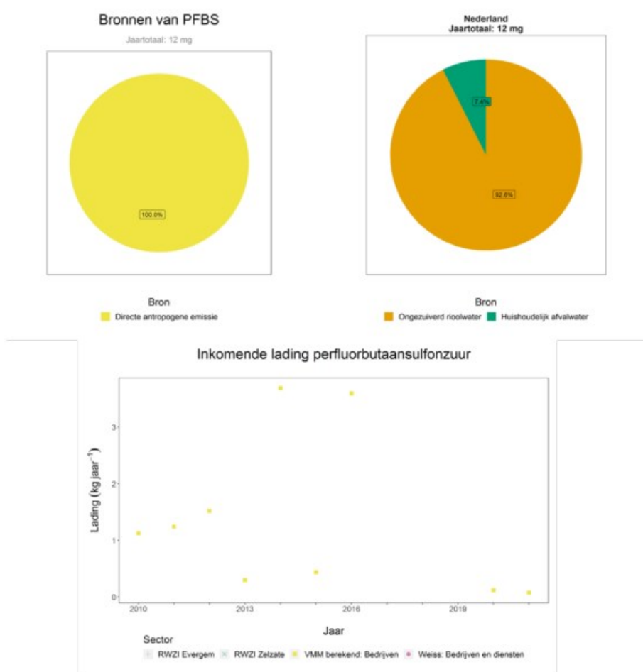
Figuur 69: PFBS – emissie naar KGT: de gemiddelde jaarlijkse lading naar het volledige kanaal (LINKSBOVEN), detail van de Directe antropogene emissie voor Nederland (RECHTSBOVEN) en de door de VMM berekende vrachten voor de bedrijven (ONDER).
