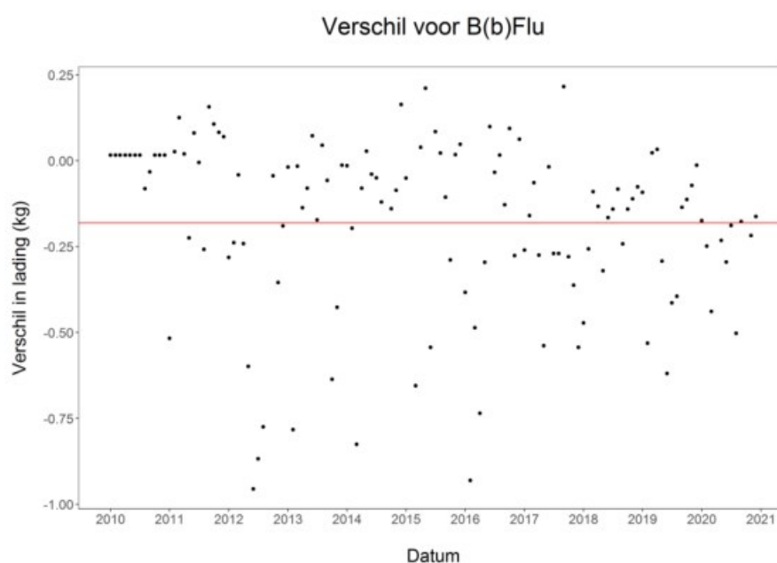
Figuur 53: B(b)F – Verschil tussen de berekende maandelijkse emissie naar het KGT en het uit de gemeten concentratie geschatte totaalgewicht aanwezig in KGT tijdens dezelfde maand (Zwarte punten). De rode lijn geeft de gemiddelde bias weer over alle punten.
