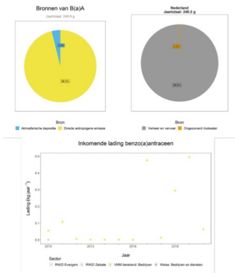
Figuur 46: B(a)A – emissie naar KGT: de gemiddelde jaarlijkse lading naar het volledige kanaal (LINKSBOVEN), detail van de Directe antropogene emissie voor Nederland (RECHTSBOVEN) en een vergelijking tussen het WEISS-model en de door de VMM berekende vrachten voor de bedrijven (ONDER).
