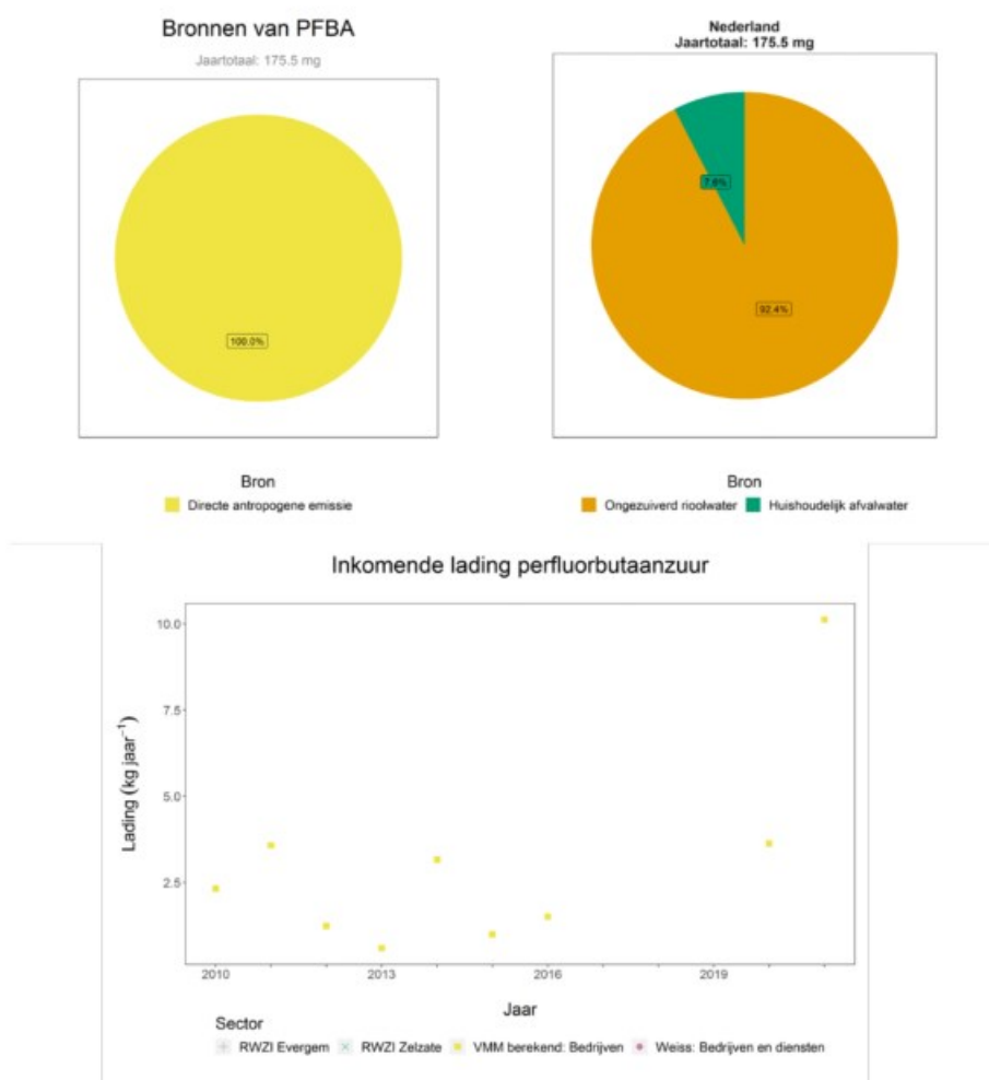
Figuur 56: PFBA – emissie naar KGT: de gemiddelde jaarlijkse lading naar het volledige kanaal (LINKSBOVEN), detail van de Directe antropogene emissie voor Nederland (RECHTSBOVEN) en de door de VMM berekende vrachten voor de bedrijven (ONDER).
