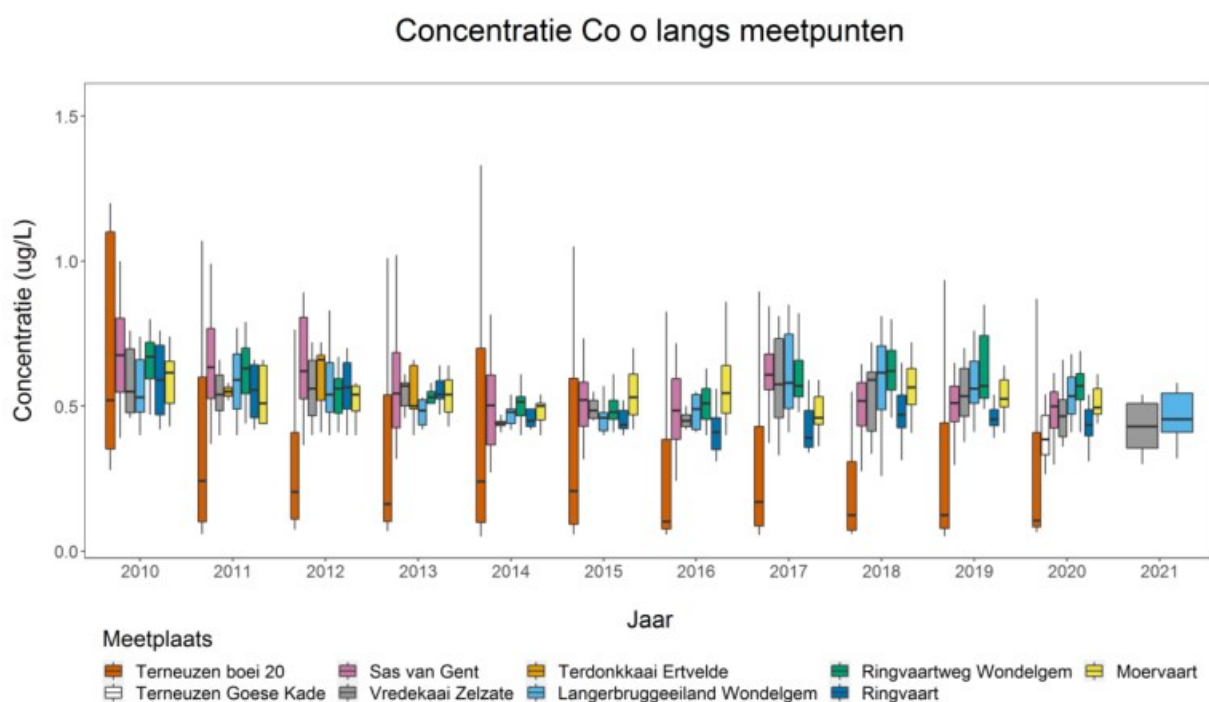
Figuur 26: Kobalt Opgelost – Verloop gemeten concentratie doorheen studiegebied.
