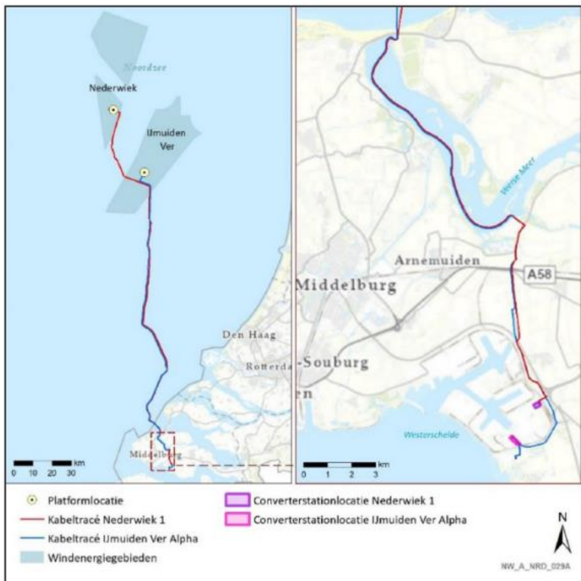
Figuur 2.3. Overzicht kabeltracé Net op zee Nederwiek 1 en parallele ligging van Net op zee IJmuiden Ver Alpha (globaal gezien wordt het inpassingsplangebied gevormd door het rode kabeltracé op de rechteraftbeelding samen met de paarse converterstationslocatie)
