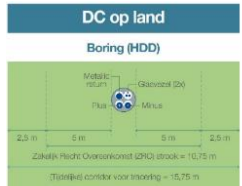
Figuur 2.9. Kabelconfiguratie boring
