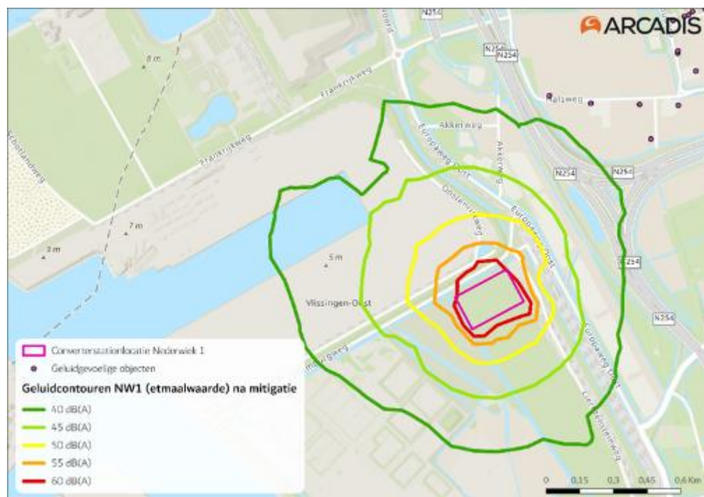
Figuur 5.13 geluidcontouren (Letmaal) vanwege het converterstation na mitigerende maatregelen
