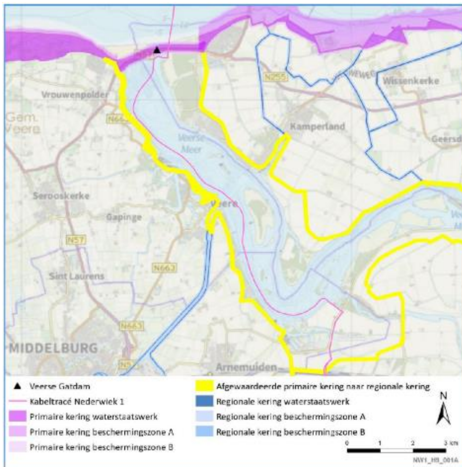
Figuur 5.19. Primaire waterkeringen rondom het Veerse Meer
