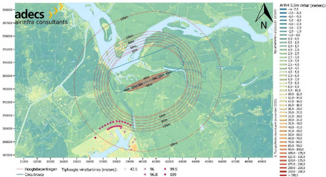
Figuur 2 Obstacle clearance areas (OCAA) na de baanrotatie i.c.m. AHN4 en windturbines.
