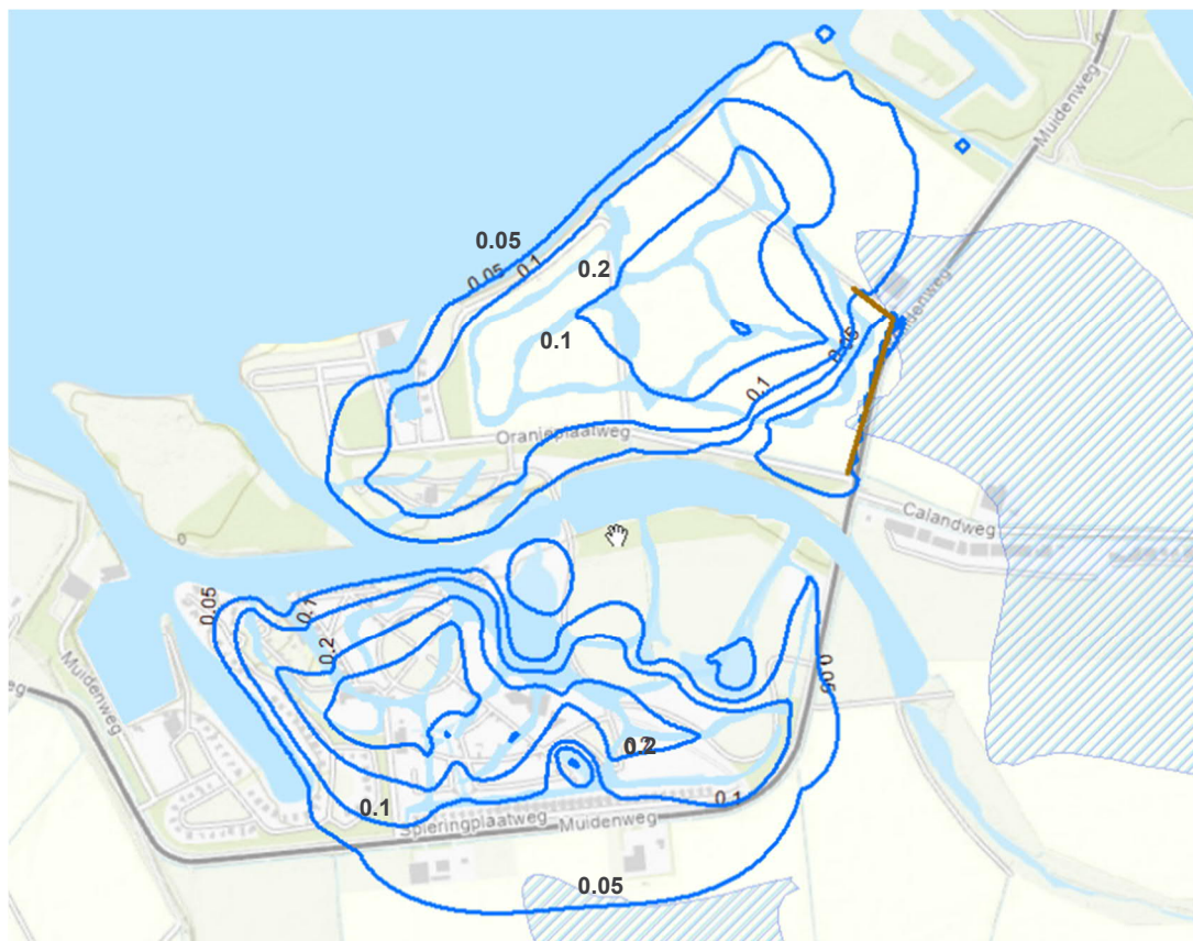
Figuur 4.4 Invloedsgebied met verticaal scherm in noordoostelijke zijde (bruine lijn). zoetwatervoorcomens zijn blauw gearceerd.
