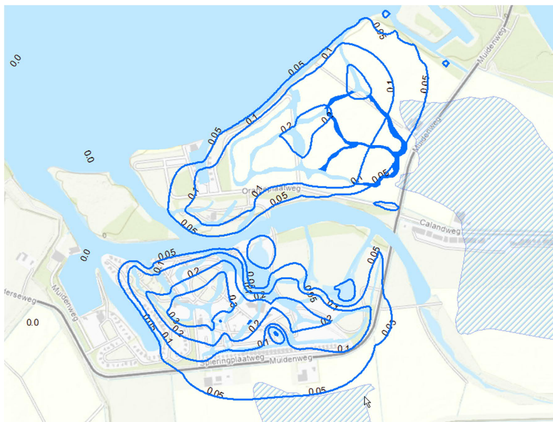
Figuur 4.6 Invloedsgebied bij folie onder noordelijke krekken (donker gearceerd). zoetwatervoorkomens zijn blauw gearceerd.
