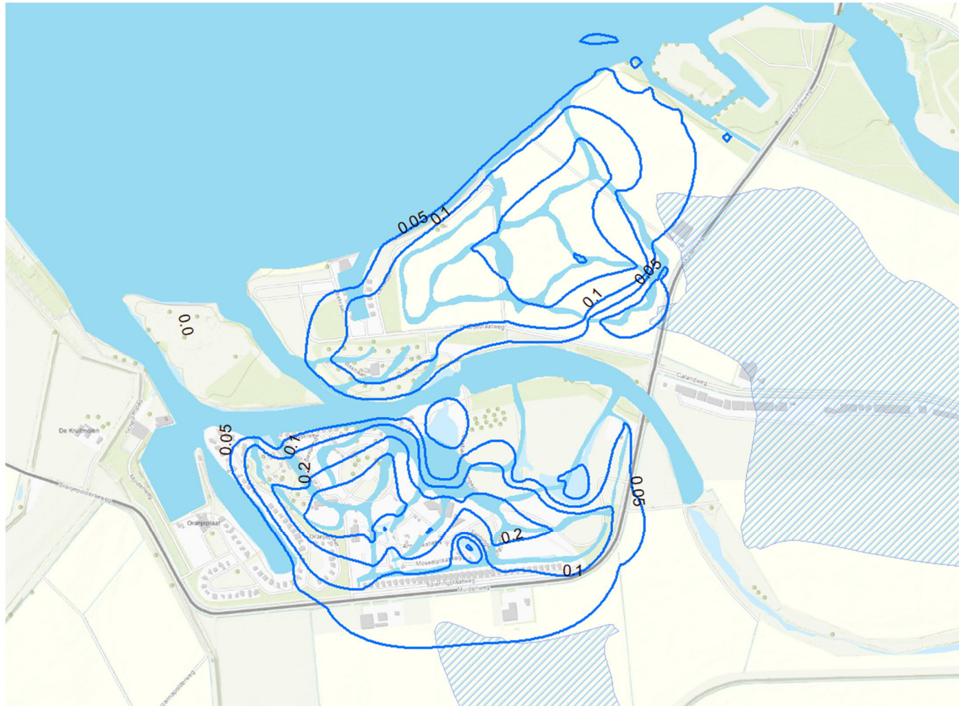
Figuur B2.3 Invloed aanleg oppervlaktewatersysteem met bodemweerstand 10 dagen (zoetwatervoorkomens zijn gearceerd)
