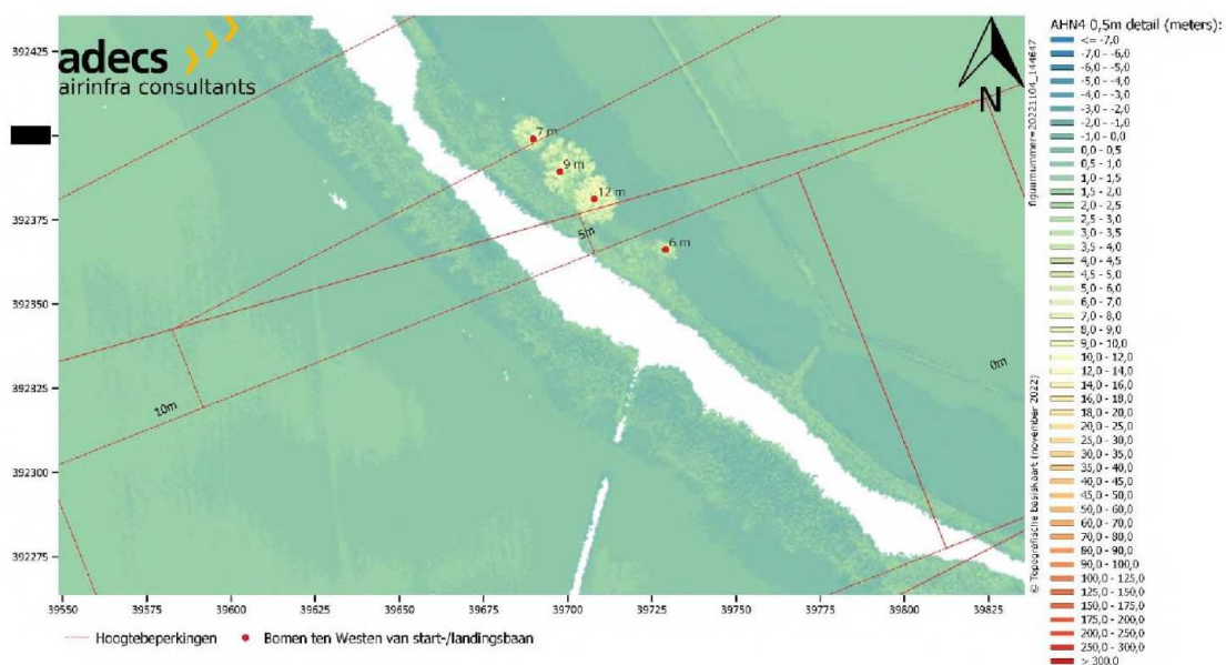
Figuur 4 Uitvergrande weergave obstakelbeperkingsvlak i.c.m. AHN4 aan westzijde start- en landingsbaan vliegveld Midden-Zeeland.
