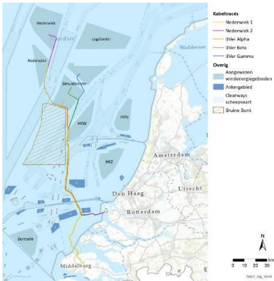
Figuur 2.2. Parallellegging Netten op zee Nederwiek 1 en 2 met Netten op zee IJmuiden Ver Alpha, Beta en Gamma
