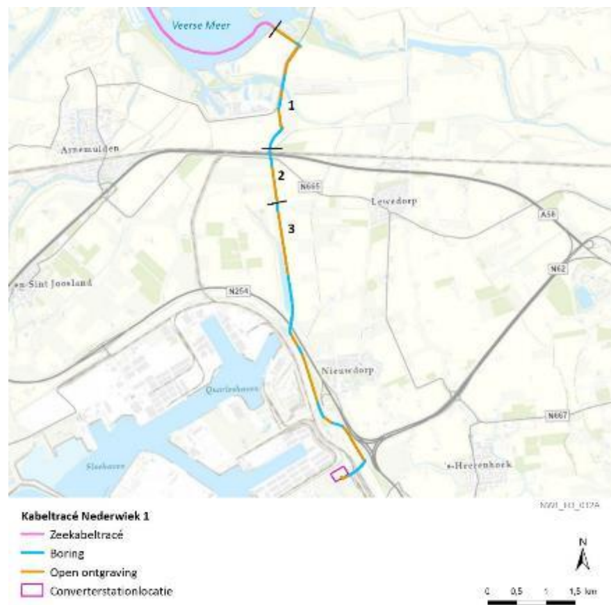
Figuur 4.4. Deeltrajecten ten zuiden van het Veerse Meer:
