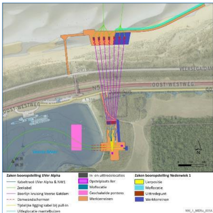
Figuur 5.18. Bovenanzicht horizontaal gestuurde boringen met de kruising Veerse Gatdam met de boring voor Net op zee IJmuiden Ver Alpha en Net op zee Nederwiek 1
