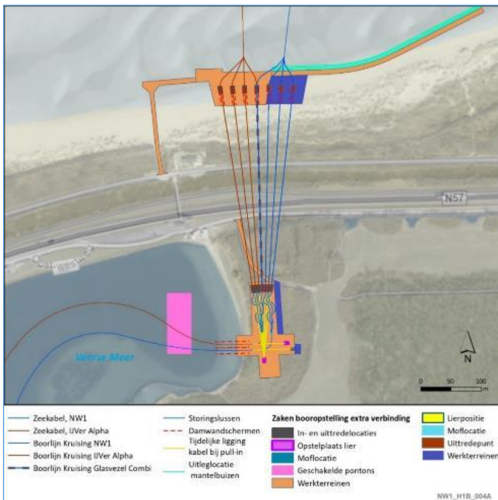
Figuur 2.5. Indicatie kruising Veeerse Gatdam IJmuiden Ver Alpha en Nederwiek 1
