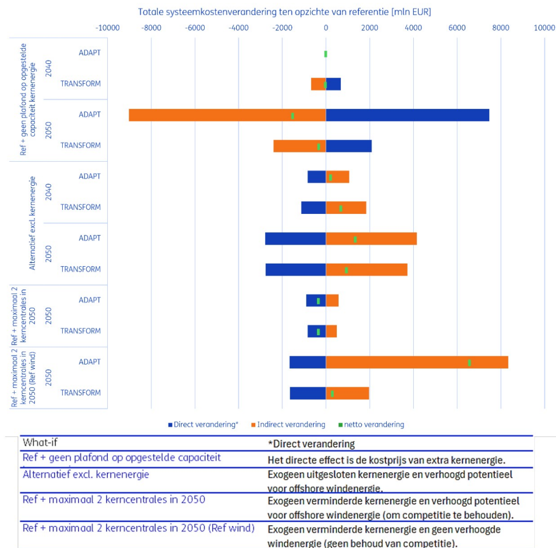
Figuur 4.2: Systeemkosten in vergelijking met de referentie bij verschillende aantallen kerncentrales. De effecten worden onderverdeeld in directe en indirecte effecten.
