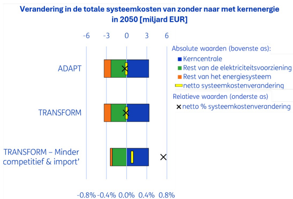
Figuur S.1: Tornadograafiek van de verandering in totale energiesysteemkosten door het toevoegen van 4 kerncentrales aan het scenario zonder kernenergie in 2050. Drie toekomstige scenario's voor Nederland: ADAPT (onder meer: meer fossiel en groter CCS-potentieel, grotere zware industrie, voortzetting huidige leefstijl), TRANSFORM (meer hernieuwbaar, strikter in gebruik fossiel en CCS, iets kleinere industrie) en TRANSFORM – Minder competitief & meer import (industriële productie staal, chemie, raffinage en kunstmest daalt met ca. 50%, import van halffabricaten toegestaan).
