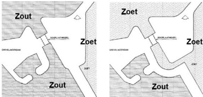
Figuur 3. Tekening uit de Driemaandelijks Berichten van de Deltawerken, uitgave 79, februari 1976. De Flakkeesse Spuisluis is bewust dicht tegen de Philipsdam aan geplaatst, om de mogelijkheid van een zoet Grevelingen open te houden. “In ieder geval zal er tot 1986 naar gestreefd moeten worden het Grevelingenmeer zo goed mogelijk zout te houden. Of het na 1986 zout zal blijven of zoet moet worden, hoeft nu nog niet te worden beslist.” (Pagina 268/508).
