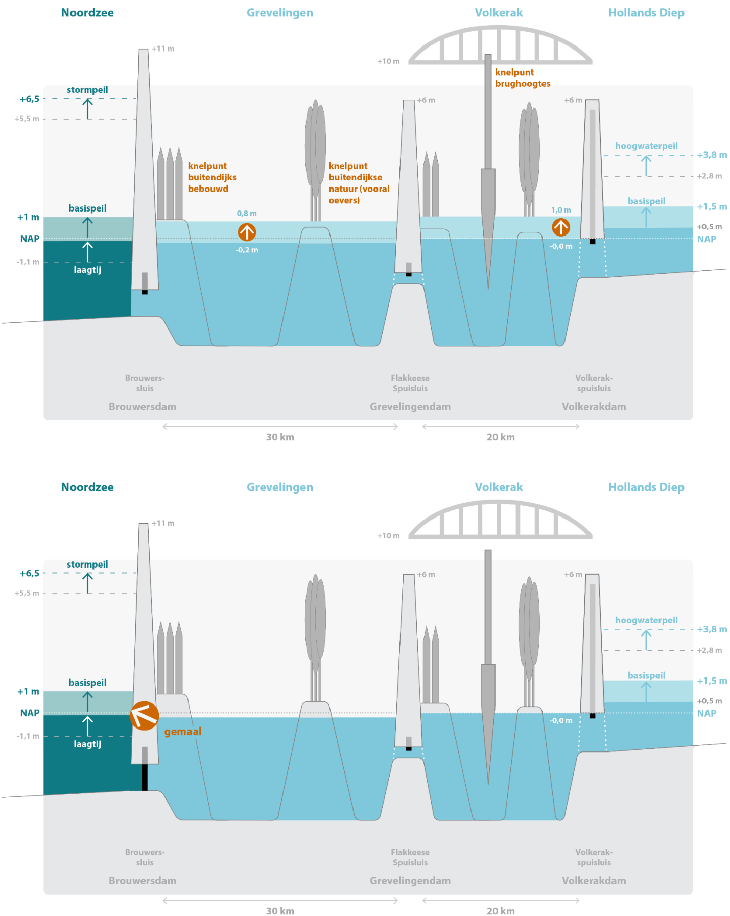
Figuur 11A en 11B. Als de zee stijgt, zijn er voor een zoet Grevelingen en het Volkerak-Zoommeer twee mogelijkheden: meestijgen, of bemalen. Alléén bemalen van het Volkerak en meestijgen van de Grevelingen ligt niet voor de hand. Voor het gemak is in deze tekening 1 meter zeespiegelstijging in 2100 gekozen. De pijlen geven de zeespiegelstijging aan.
