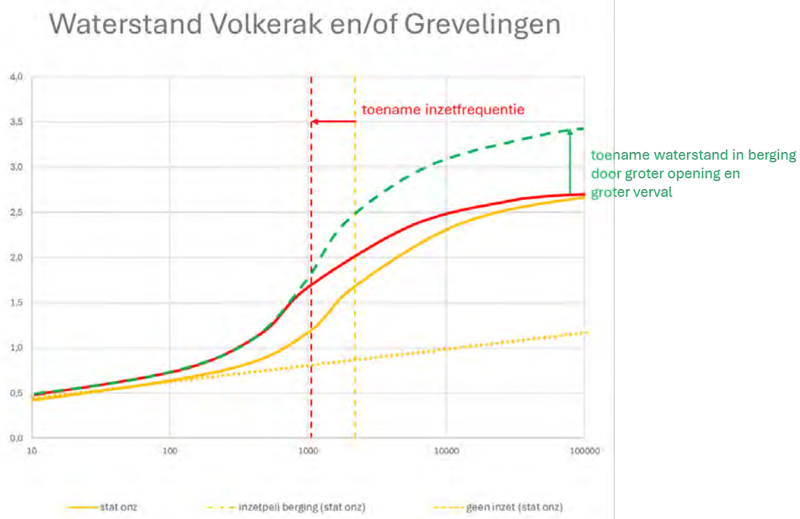
Figuur 27: Schets wijziging waterstand op het Volkerak en/of de Grevelingen door een toename van inzetfrequentie en een toename van de waterstand na inzet.
