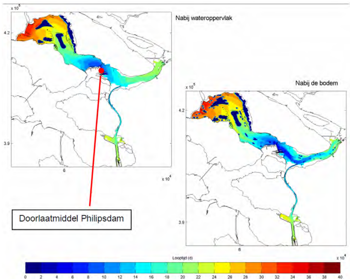
Figuur 6: Gemiddelde looptijd in dagen van zout water uit de Oosterschelde dat ingelaten wordt in een open verbonden zout Grevelingen-Krammer-Volkerak via een fictief doorlaatmiddel in de Philipsdam aangegeven met de rode stip. Figuur is afkomstig uit Deltares (2008).
