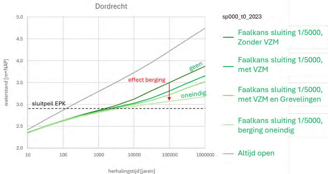
Figuur 26: Waterstandfrequentie te Dordrecht in 2023 voor 5 berekeningen: (1) EPK 1/5000 zonder waterberging, (2) EPK 1/5000 plus waterberging VZM, (3) EPK 1/5000 plus waterberging VZM + Grevelingen, (4) EPK 1/5000 plus theoretisch oneindige berging en (5) EPK sluit niet plus waterberging wordt niet ingezet
