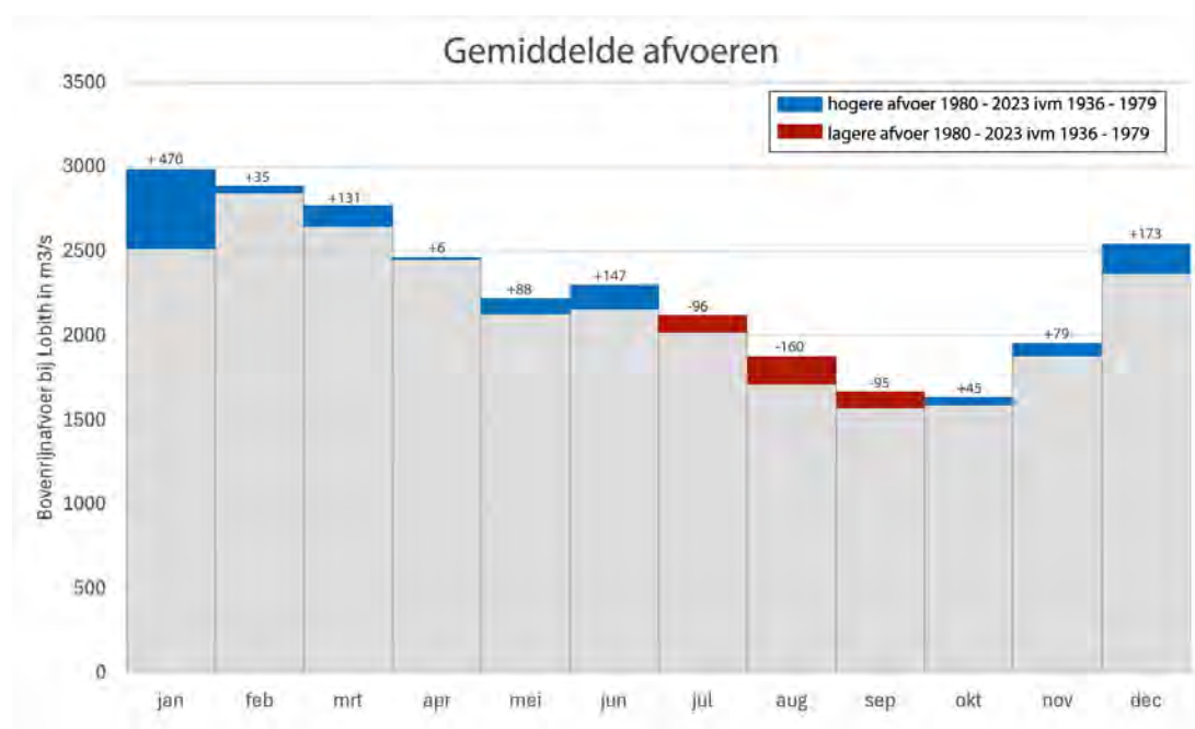
Figuur 13: Gemiddelde afvoeren van de Rijn bij Lobith over de periode 1936-2023. Figuur afkomstig van https://www.waterpeilen.nl/berichten/rivierafvoeren-blijven-voorlopig-hoog-voor-de-tijd-van-het-jaar .
