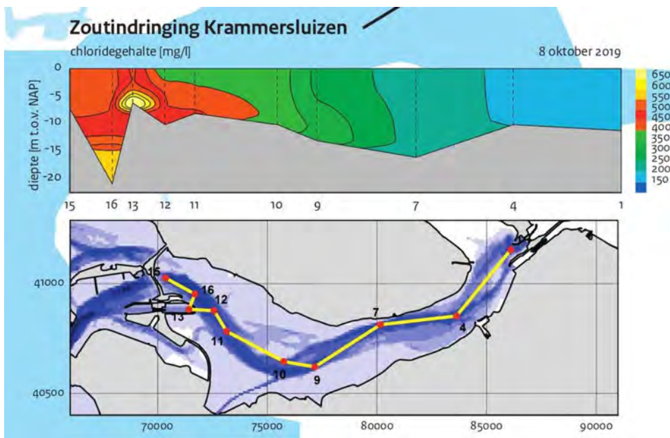
Figuur 11: Zoutindringing bij de Krammersluizen. Figuur afkomstig van de Infographic Operationeel Watermanagement Volkerak-Zoommeer ( https://www.deltaexpertise.nl/wiki/index.php/Infographic_Volkerak-Zoommeer_VN ).
