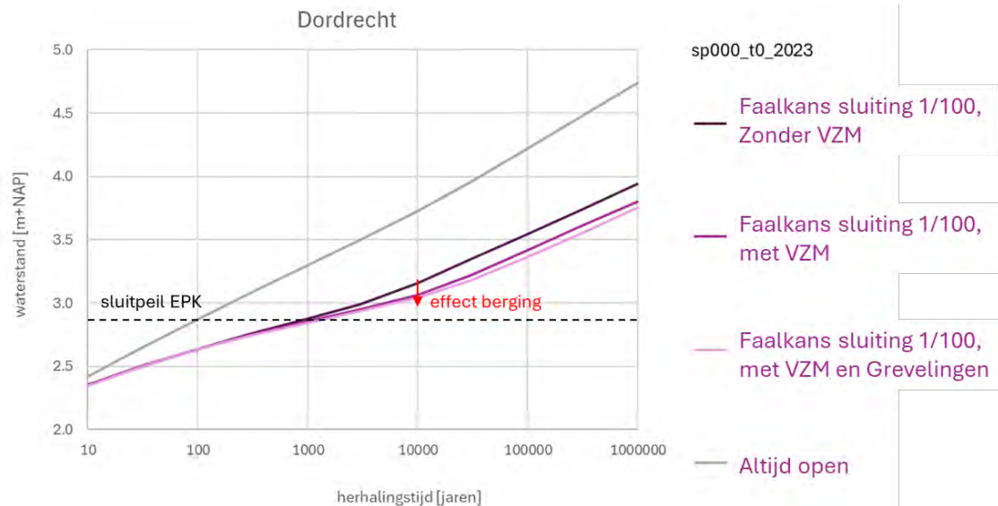
Figuur 23: Waterstandfrequentie te Dordrecht in 2023 voor vier berekeningen: (1: donkerpaarse lijn) Europoortkering 1/100 zonder waterberging VZM, (2: middelste paarse lijn) Europoortkering 1/100 plus waterberging VZM, (3: lichtpaarse lijn) Europoortkering 1/100 plus waterberging VZM + Grevelingen en (4) Europoortkering sluit niet, geen inzet waterberging (grijze lijn).
