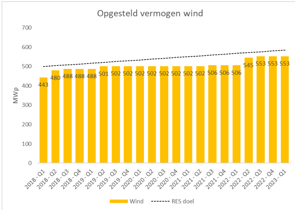
Figuur 2 1 : Ontwikkeling opgesteld en aangesloten vermogen windenergie MWP (bron: Stedin)
