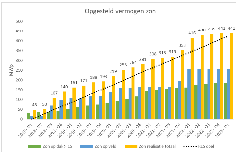
Figuur 3: Ontwikkeling opgesteld en aangesloten vermogen Zon MWP (bron: Stedin)
