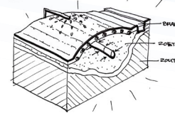
KREEKRIJFILTIRATIE
