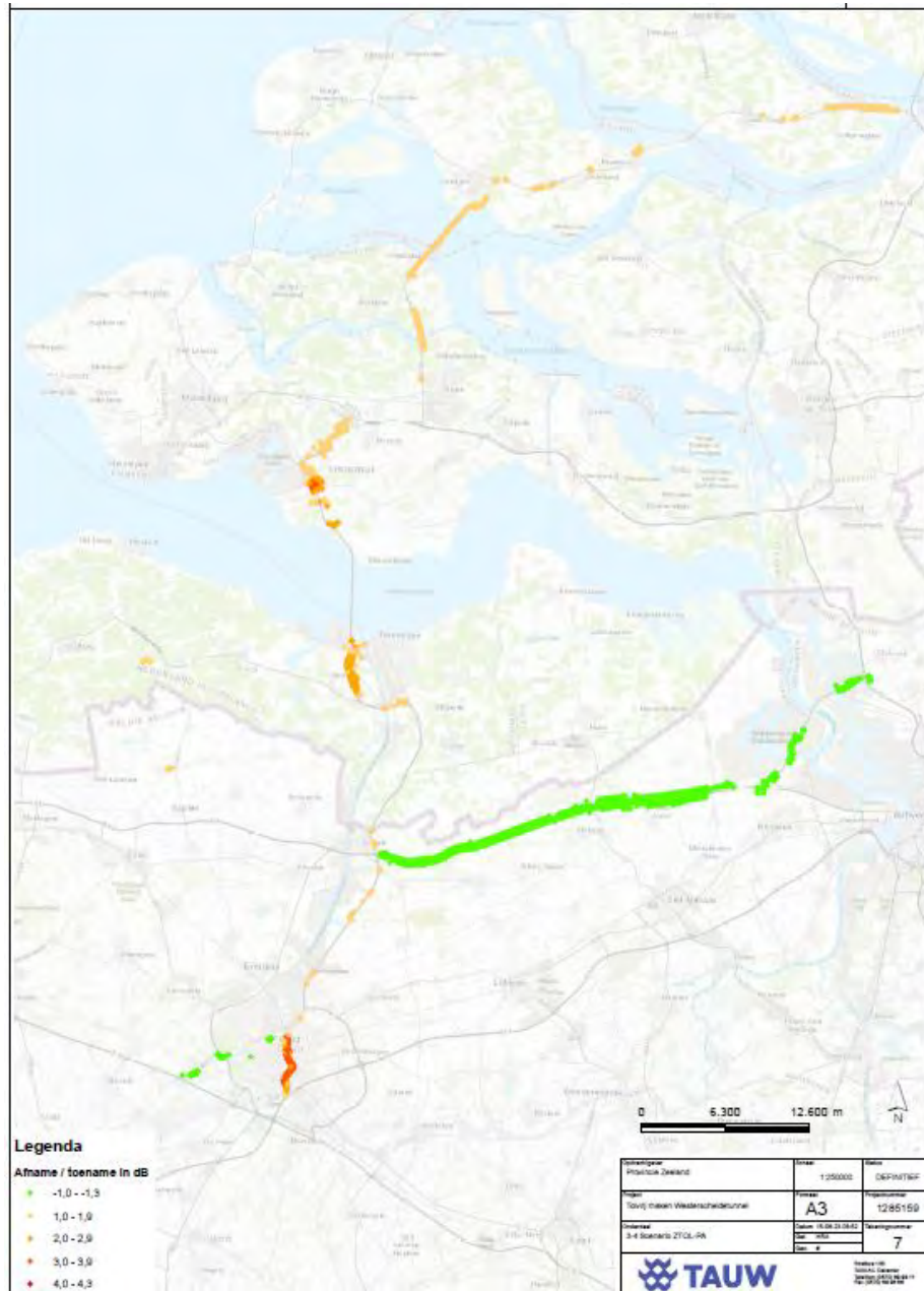
Figuur 5.4 Toe- en afnames \geq 1,0 dB voor scenario 2033 zonder tol voor zowel personenauto's als vrachtwagens met maximum snelheid 100 km/uur (ZTOL)
