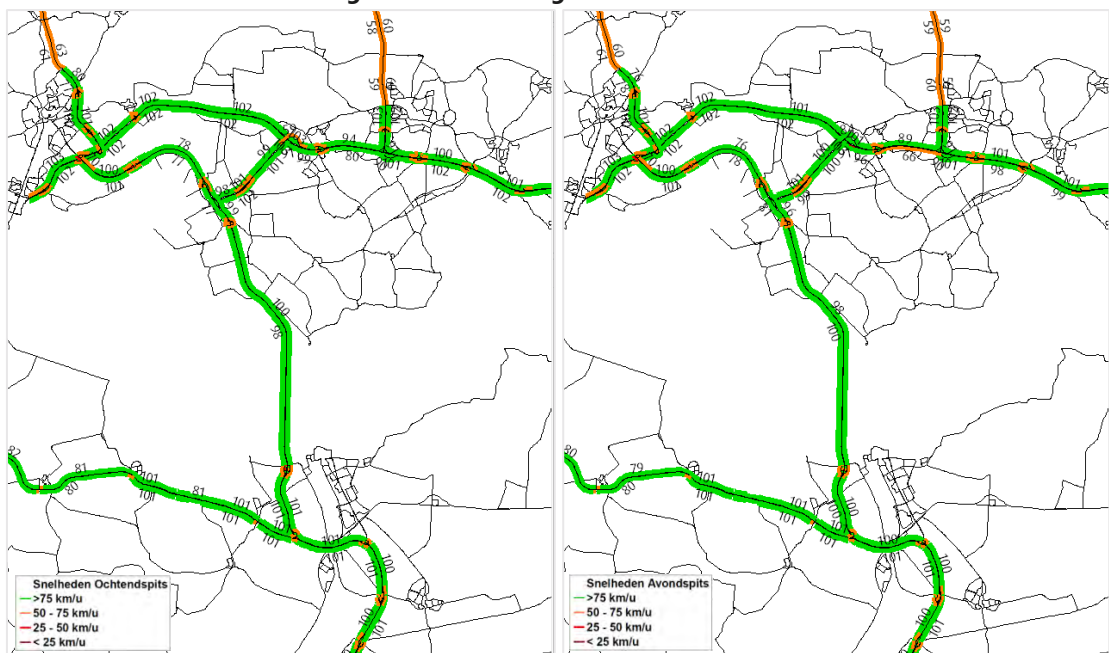
Figuur 5.24: Rijksnelheden in de ochtend- en avondspits Alternatief 2030 tol vrij scenario Hoog
