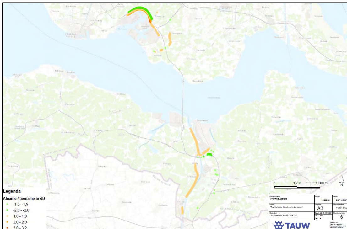
Figuur 5.3 Toe- en afnames \geq 1,0 dB voor scenario 2023 zonder tol voor personenauto's en met tol vrachtwagens met maximum snelheid 80 km/uur (80SPD_VRTOL)
