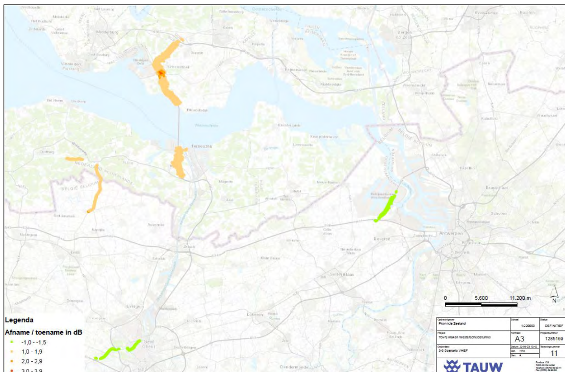
Figuur 5.6 Toe- en afnames \geq 1,0 dB voor scenario 2033 zonder tol voor zowel personenauto's als vrachtwagens met vrachtwagenheffing en maximum snelheid 100 km/uur (VHEF)
