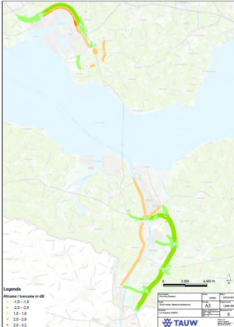
Figuur 5.2 Toe- en afnames \geq 1,0 dB voor scenario 2023 zonder tol voor zowel personenauto's als vrachtwagens met maximum snelheid 80 km/uur (80SPD)
