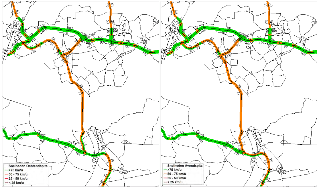
Figuur 5.29: Rij snelheden in de ochtend- en avondspits Alternatief 2030 tolvrij personenauto's en 80 km/uur scenario Hoog
