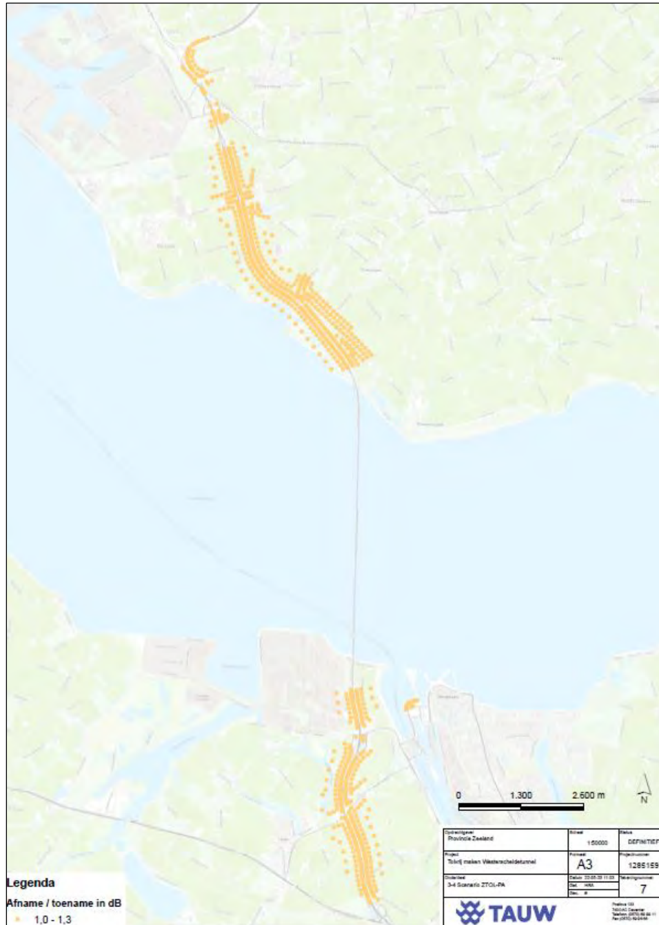
Figuur 5.7 Toe- en afnames \geq 1,0 dB voor scenario 2033 zonder tol voor personenauto's en met tol vrachtwagens met maximum snelheid 100 km/uur (ZTOL_PA)
