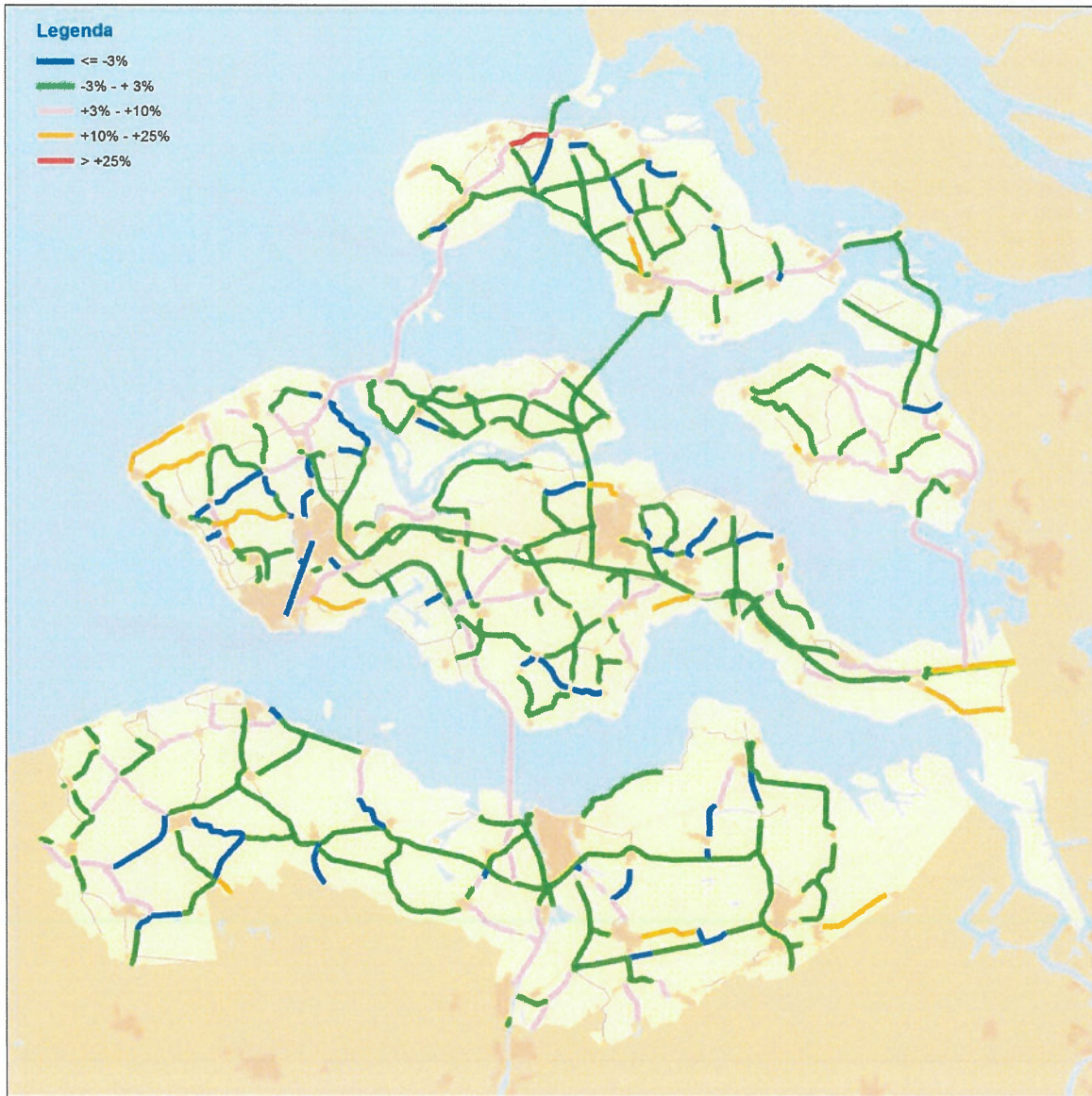
Verhouding jaargemiddelde intensiteit 2013 - 2014
