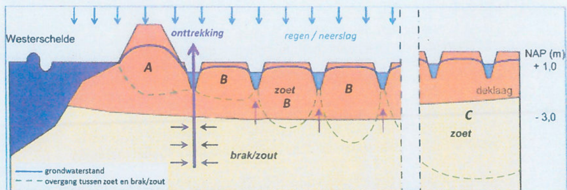
Figuur 3.4 Een impressie van een bodemopbouw met de aanwezigheid van zoetwaterlensen en een zoetwaterbel in de ondergrond (Witteveen+Bos, 2010). A en B zijn zoetwaterlensen waarvan A in de dijk ligt. C is een zoetwaterbel. De groene stippellijn is de grens tussen zoet en zout. De onttrekking wordt via het oppervlakte water afgevoerd.
