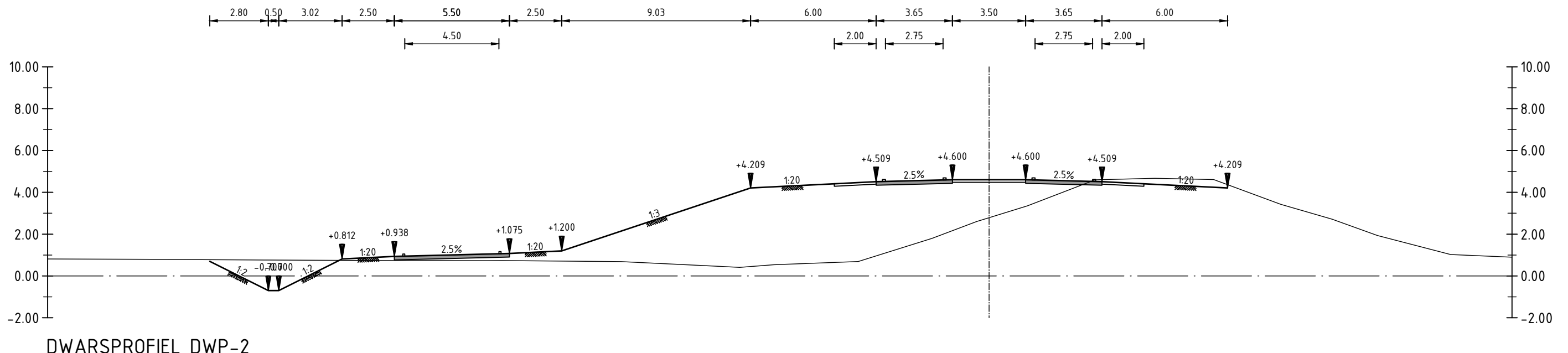
DWARSPROFIEL DWP-2 Schaal 1:200
