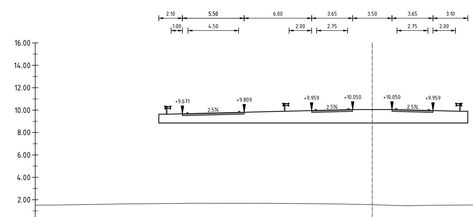
DWARSPROFIEL DWP-1 Schaal 1:200
