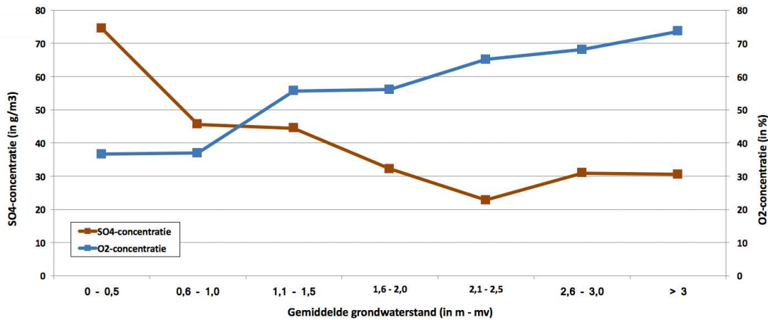
Figuur 2. Relatie tussen gemiddelde grondwaterstand en respectievelijk zuurstofconcentratie (blauwe lijn) en sulfaatconcentratie (bruine lijn) in het bovenste grondwater. Bron data: RIVM (meetdata 2010).
